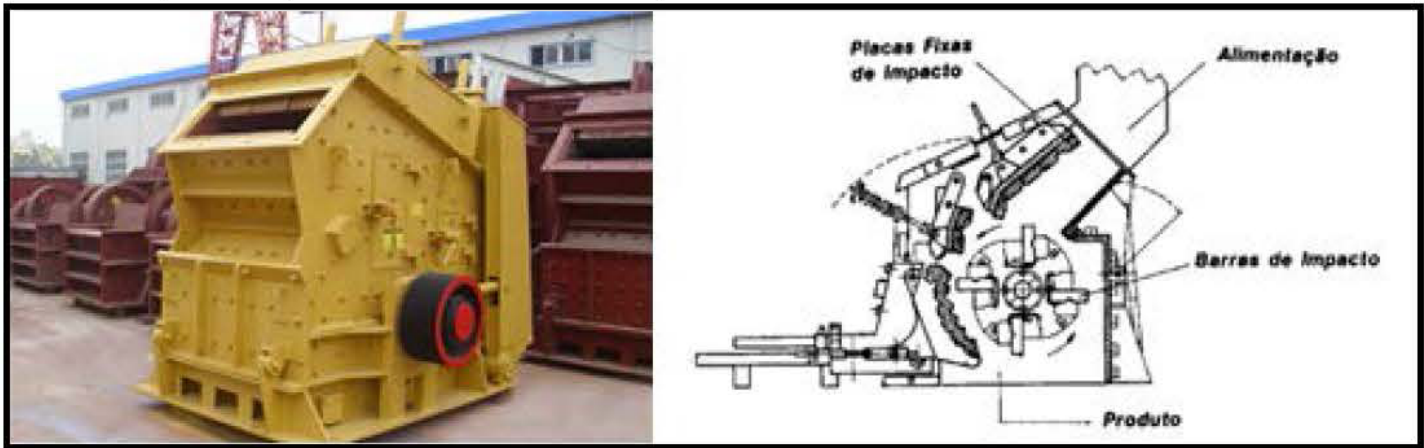
Figura 35. Exemplo e esquema de britador de impacto
