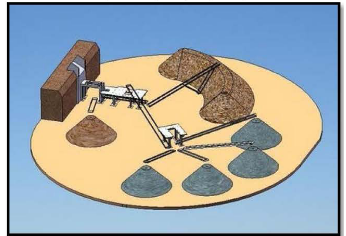
Figura 33. Esquema de URCC, com britagem e separação por tipo de resíduos e granulometria.
