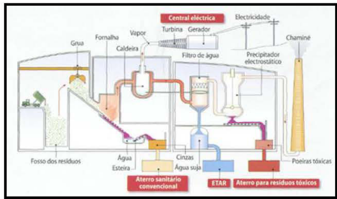
Figura 31. Funcionamento de uma central de tratamento térmico
