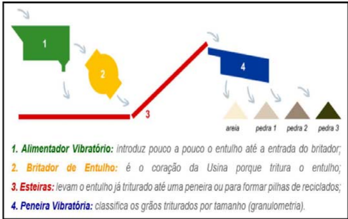
Figura 32. Fluxograma de uma usina de RCC
