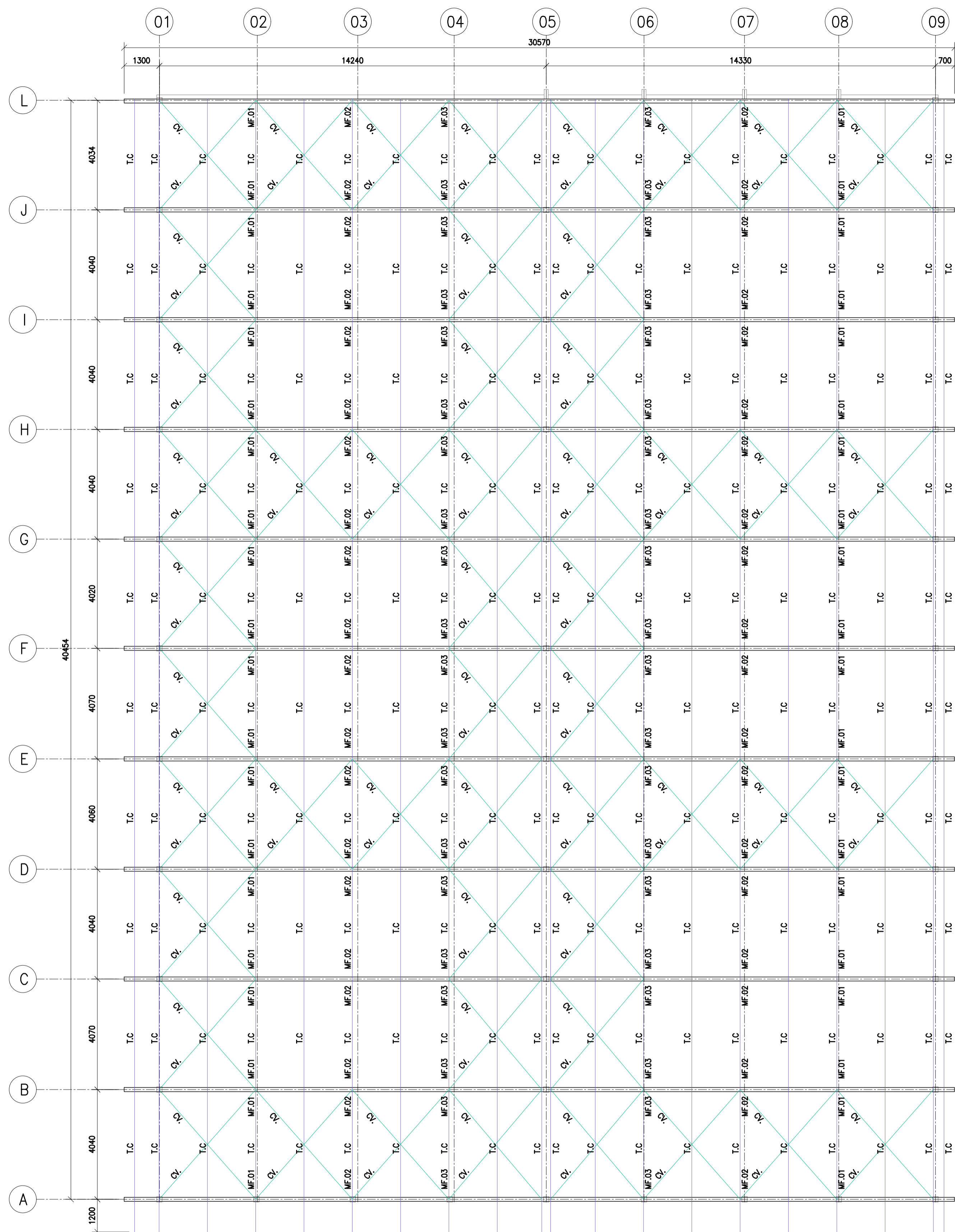
PLANTA DE LOCAÇÃO – TESOURAS, CV E MF
