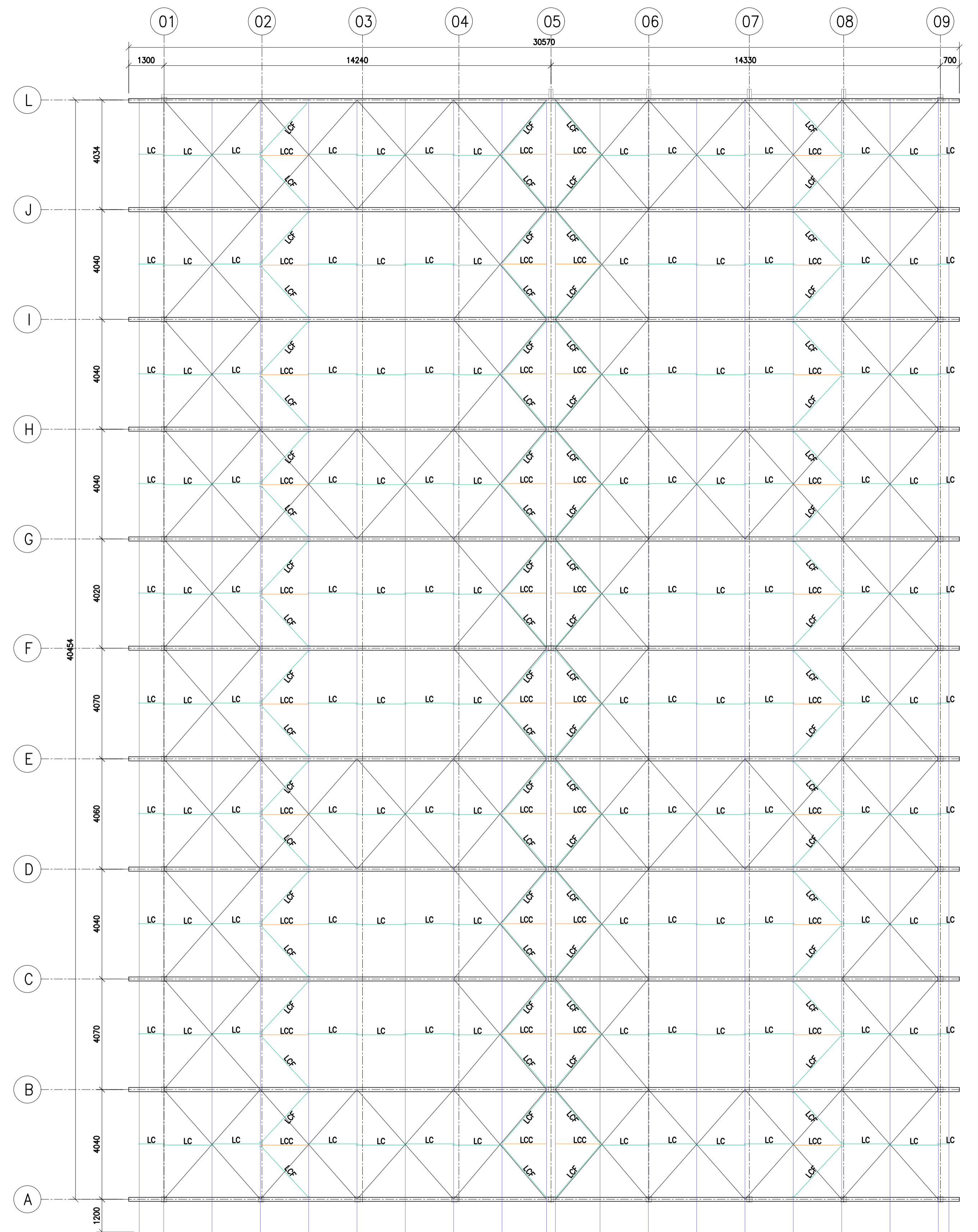
PLANTA DE LOCAÇÃO – TERÇAS, L.C, L.C.C E L.C.F
