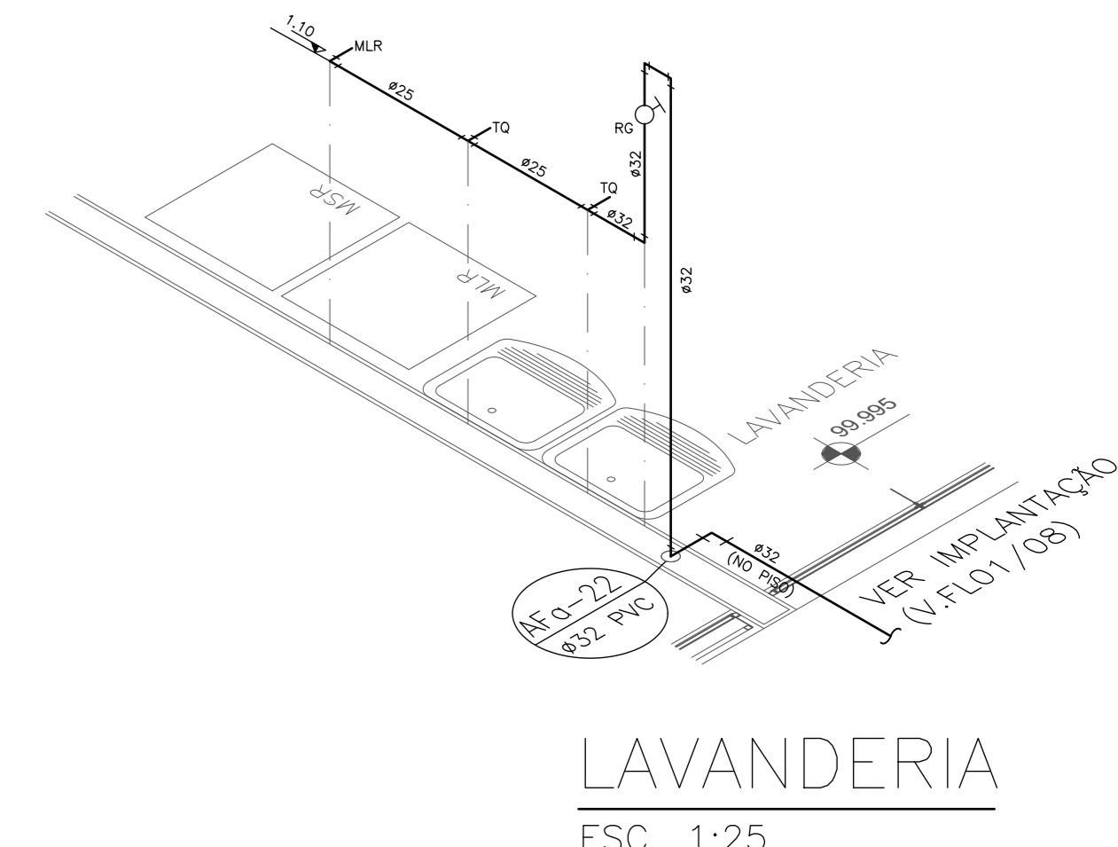
LAVANDERIA ESC. 1:25
