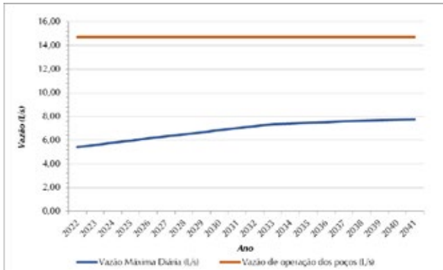
Figura 8.5 – Demandas Máximas Diárias (L/s) X Vazão de operação dos poços (L/s) – SAA Jardim Sandra
