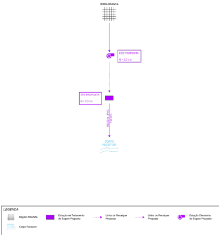
Figura 9 – Croqui do Sistema de Esgotamento Sanitário Proposto para o bairro Irara Branca.
