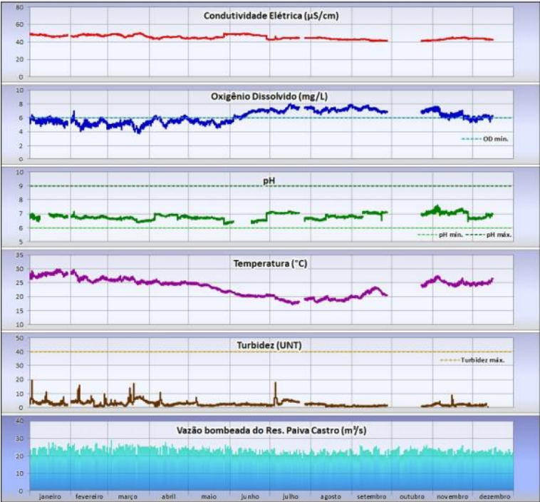
Figura 8.2 - Evolução dos parâmetros medidos pela Estação Automática Águas Claras de janeiro a dezembro de 2019 Fonte: CETESB, 2020.
