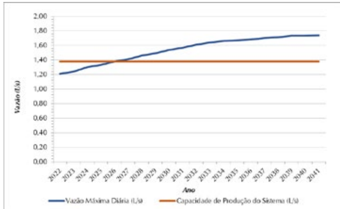
Figura 8.7 – Demandas Máximas Diárias (L/s) X Vazão de operação dos poços (L/s) – SAA Irara Branca
