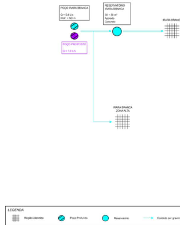
Figura 10.3 – Croqui das intervenções propostas para o sistema de abastecimento de água Irara Branca
