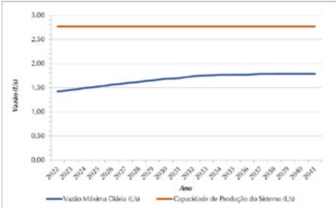
Figura 8.9 – Demandas Máximas Diárias (L/s) X Vazão de operação dos poços (L/s) – SAA Ypeville
