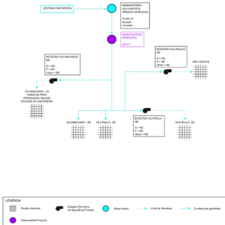
Figura 10.1 – Croqui das intervenções propostas para o sistema de abastecimento de água Vila Santista-Vila Machado
