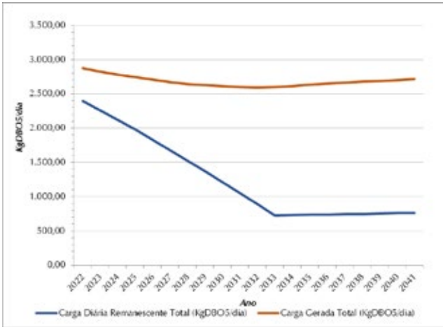
Figura 8.14 - Evolução de Cargas Orgânicas (Kg DBO 5,20 /Dia)
