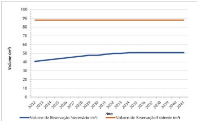
Figura 8.10 - Volume de Reservação Necessário (m³) x Volume de Reservação Atual (m³) - SAA Ypeville
