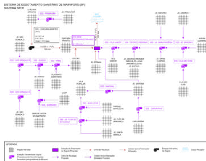
Figura 10.8 – Croqui das intervenções propostas para o sistema de esgotamento sanitário Sede
