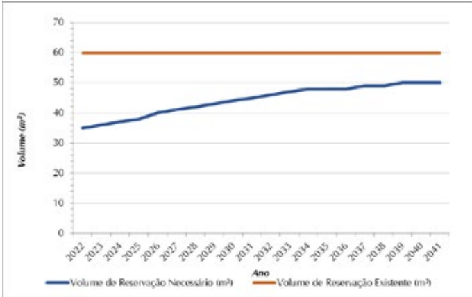
Figura 8.8 - Volume de Reservação Necessário (m³) x Volume de Reservação Atual (m³) - SAA Irara Branca Verifica-se que o SAA Irara Branca possui reservação suficiente para atender às demandas durante todo o horizonte de planejamento, uma vez que a capacidade atual da reservação do sistema é de 60 m³ e o volume de reservação necessário varia entre 35 m³ (2022) e 50 m³ (2041), ou seja, inferior ao volume instalado.
